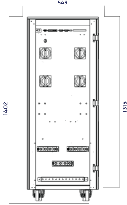
3.3.1 160kVA U2 //U3 Model Ölçüleri (mm)
