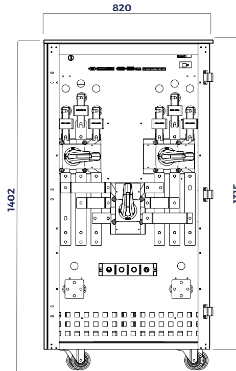
3.3.3 300kVA U2 // U3 Model Ölçüleri (mm)
