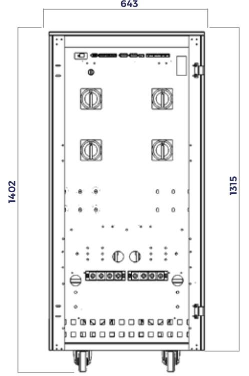
3.3.2 200 kVA U2//U3 Model Ölçüleri (mm)
